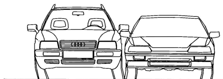
Bild 6 Trennung bei Streifkollisionen infolge: Wanken durch Ein- bzw. Ausfedern der Karosserie
