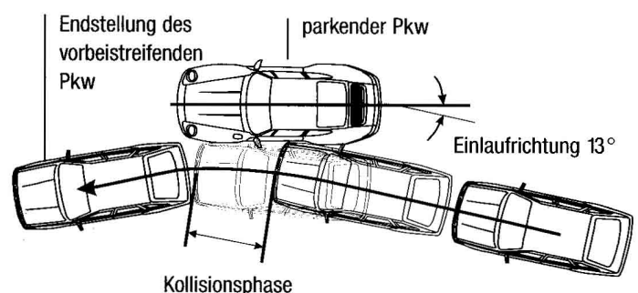
Bild 1 Ablauf einer typischen Streifkollision mit einem parkenden Fahrzeug (Modelle aus der VENUS-Fahrzeugdatenbank)
