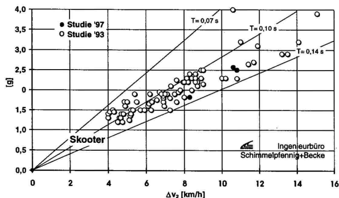
Bild 15 Meßwerte Skooter-Versuche Fig. 15 Measurement of bumper car collisions
