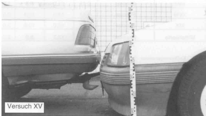
Bild 2 Unbeschädigte Versuchsfahrzeuge und Anstoßkonfiguration Fig. 2 Undamaged crash test vehicles and impact configuration
