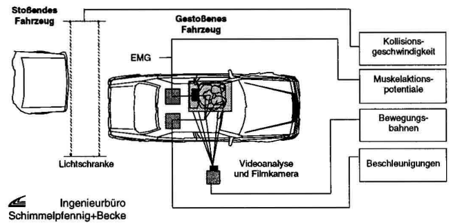
Bild 4 Versuchsaufbau Fig. 4 Experimental setup
