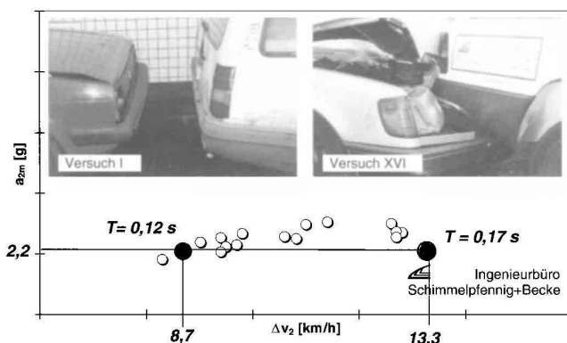
Bild 21 Kollisionsbedingte Geschwindigkeitsänderung in Abhängigkeit der massenbewerteten Differenzgeschwindigkeit Fig. 21 Change in velocity dependent on weight adjusted velocity
