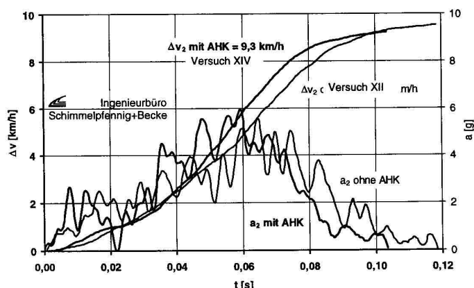
Bild 20 Meßwerte bei unterschiedlicher Kollisionsdauer Fig. 20 Measurement with different collision duration
