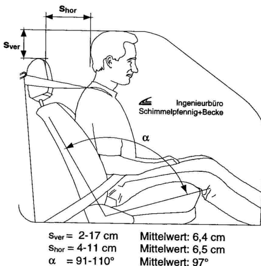
Bild 3 Ausgangsposition Fig. 3 Initial position
