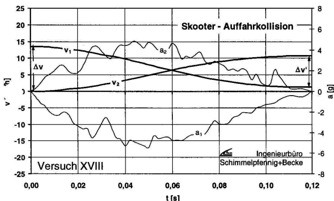
Bild 18 Skooter-Kollision Fig. 18 Bumper car collision
