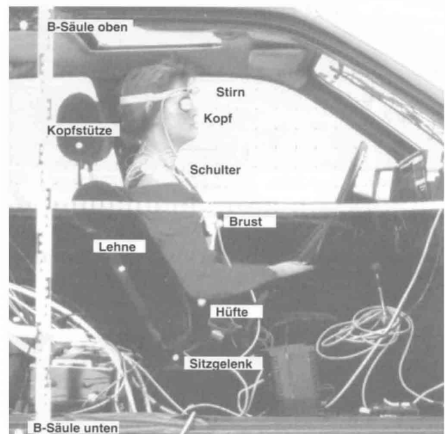
Bild 5 Markerpositionen Fig. 5 Positions of markers
