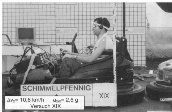
Bild 7 Versuchsaufbau Autoskooter-Versuch Fig. 7 Experimental setup of bumper car crash tests
