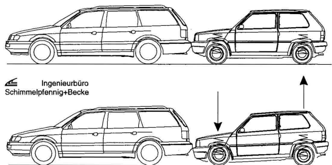
Bild 11 Höhenzuordnung in Abhängigkeit des Bremszustandes Fig. 11 Vertical offset dependent on brake conditions
