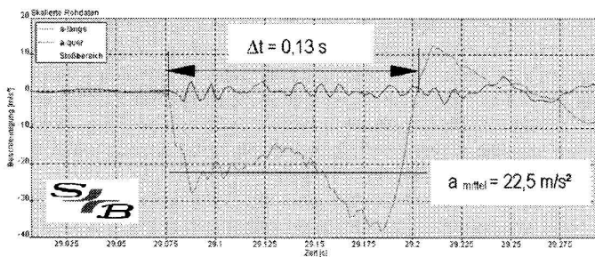
Bild 6 Beschleunigungsverlauf Fig. 6 Course of acceleration
